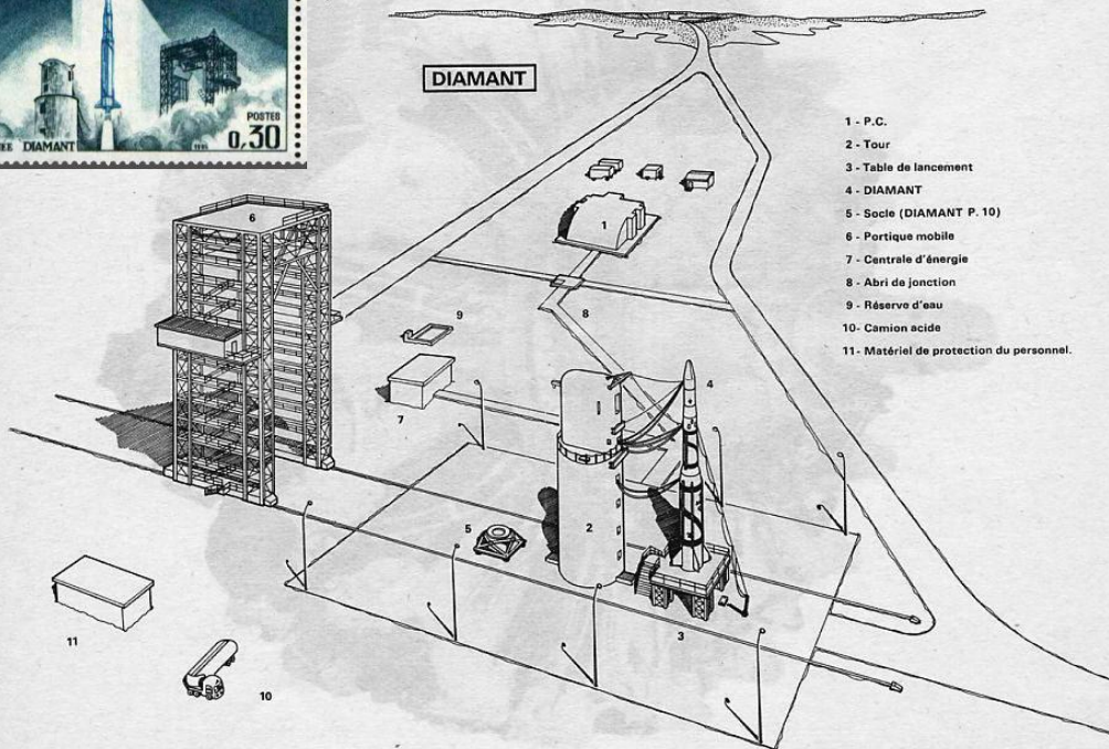
Schéma d'installation de la fusée Diamant
